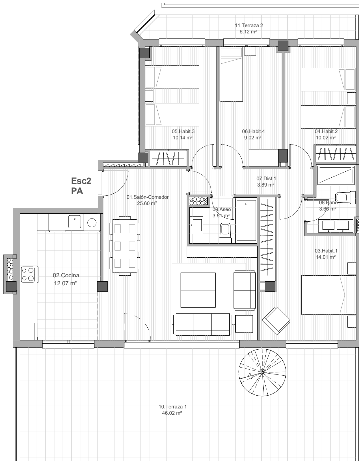
1 V_Planta Atico_Esc2 PA V19 1 : 75
